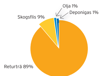
Bränslemix Nyköping 2008
