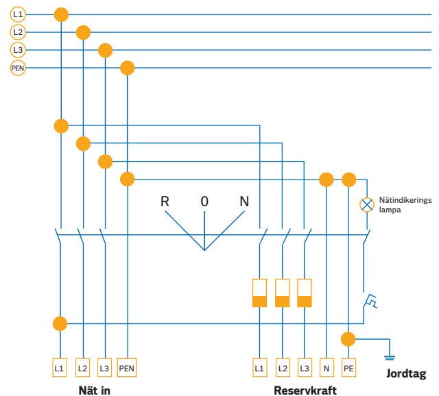
Figur 6 Reservkraft TN-C
