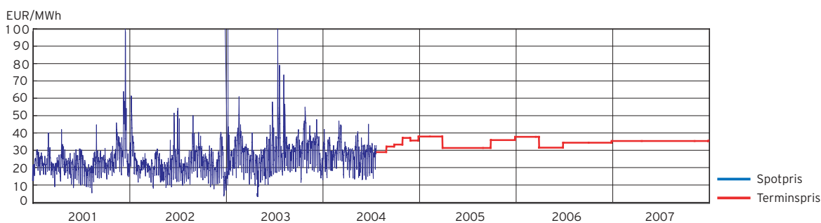
Tyska elpriser 2000-2007
