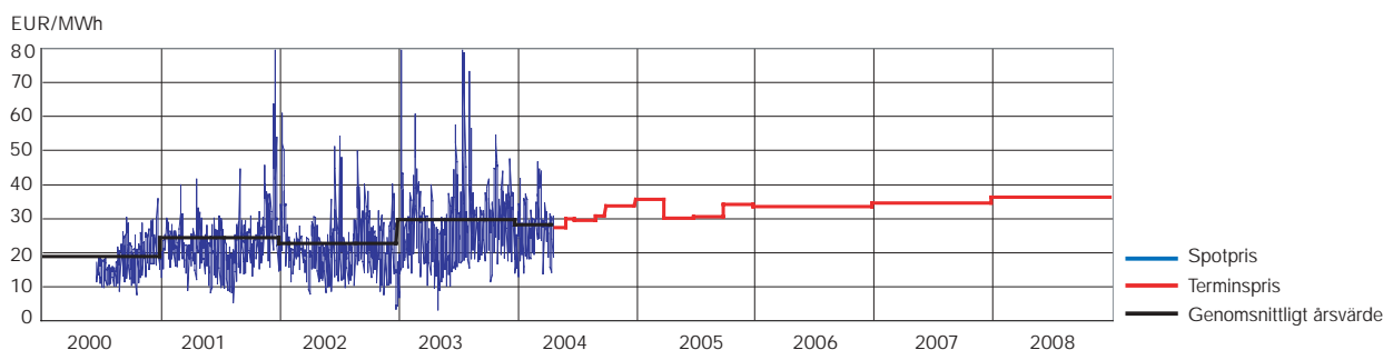
Tyska elpriser 2000–2008
